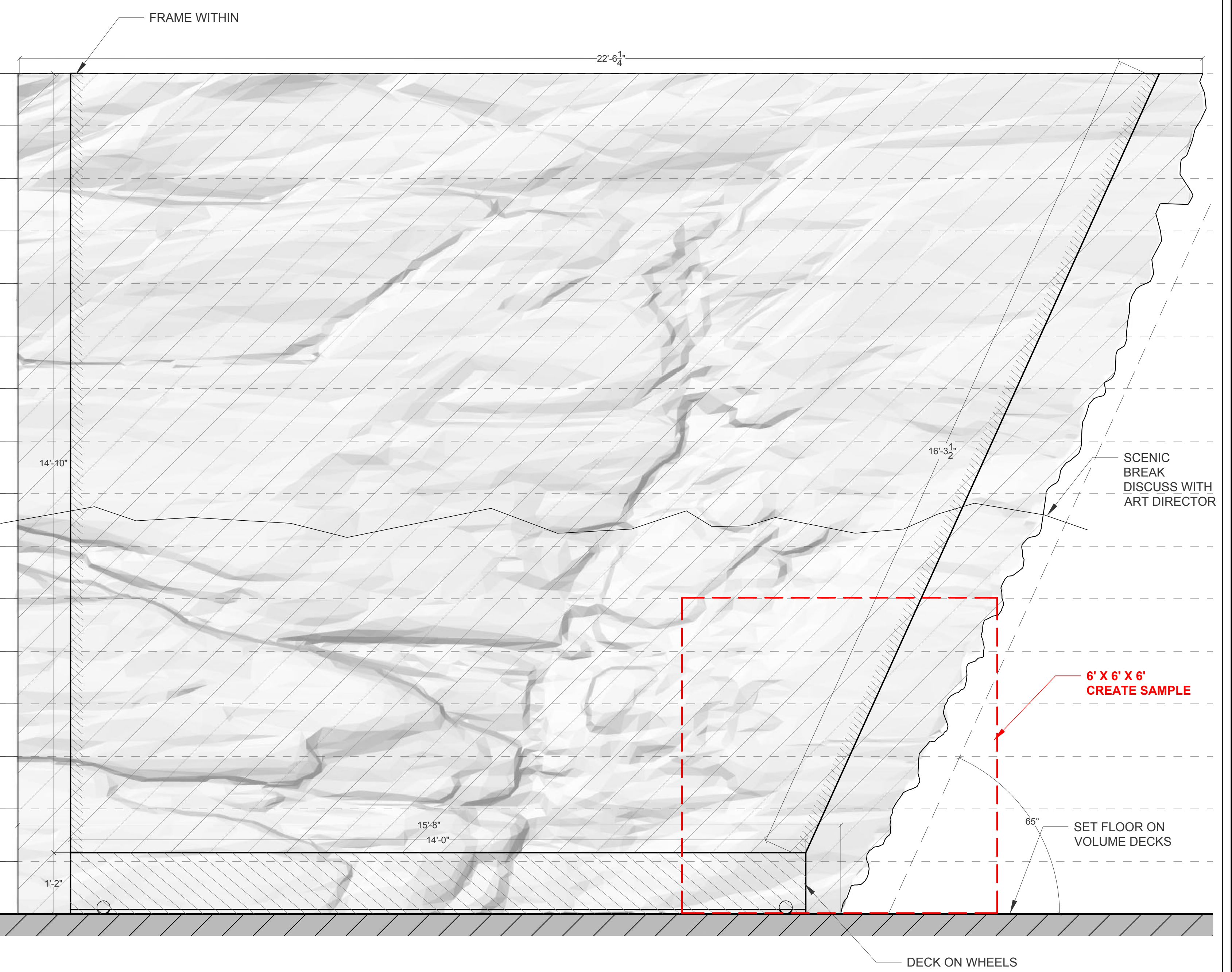
S1 04 SECTION 1 - PILLAR A SCALE: \frac{3}{4}'' = 1'-0''
