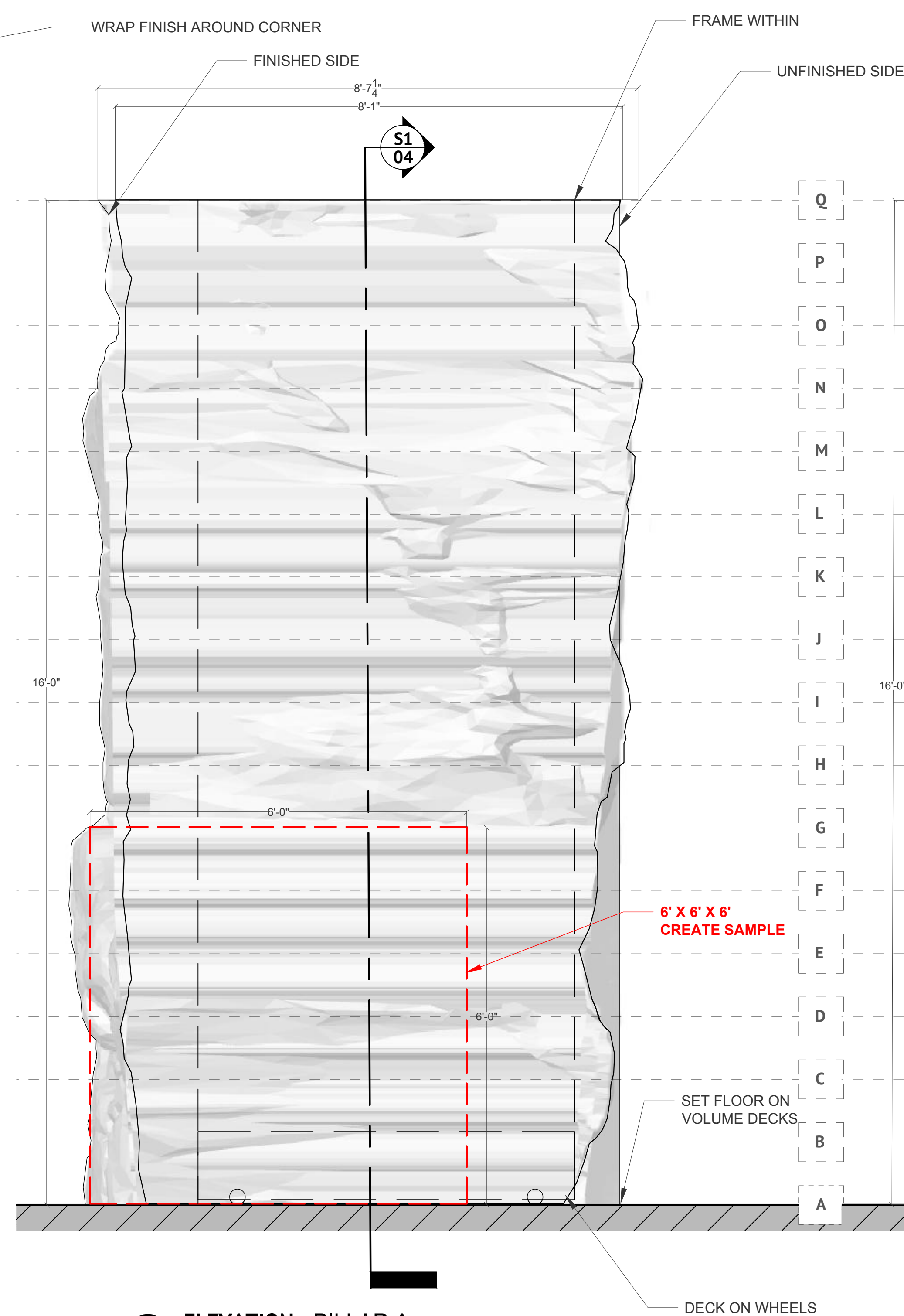
A ELEVATION - PILLAR A SCALE: \frac{3}{4}'' = 1'-0''
